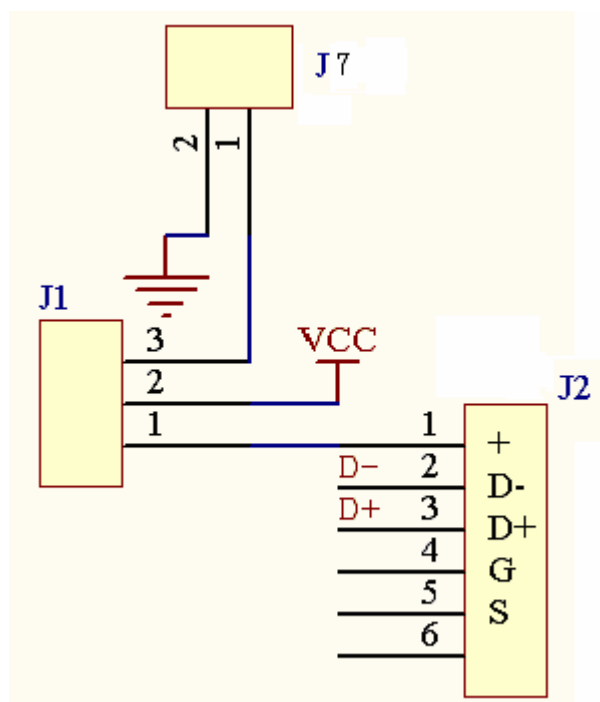
图 6 数字电源的接线原理
