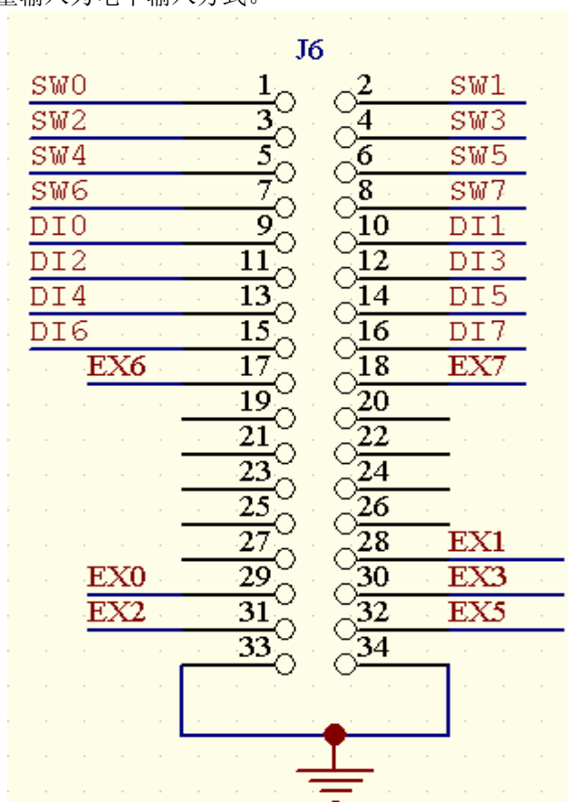
图3 第一组8通道开关量输入与8通道开关量输出接线图
