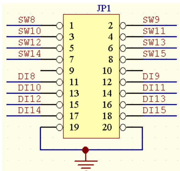
图4 第二组8路开关量输入与开关量输出定义
