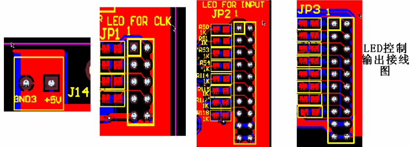
图 7 40 通道 LED 开关量控制输出
