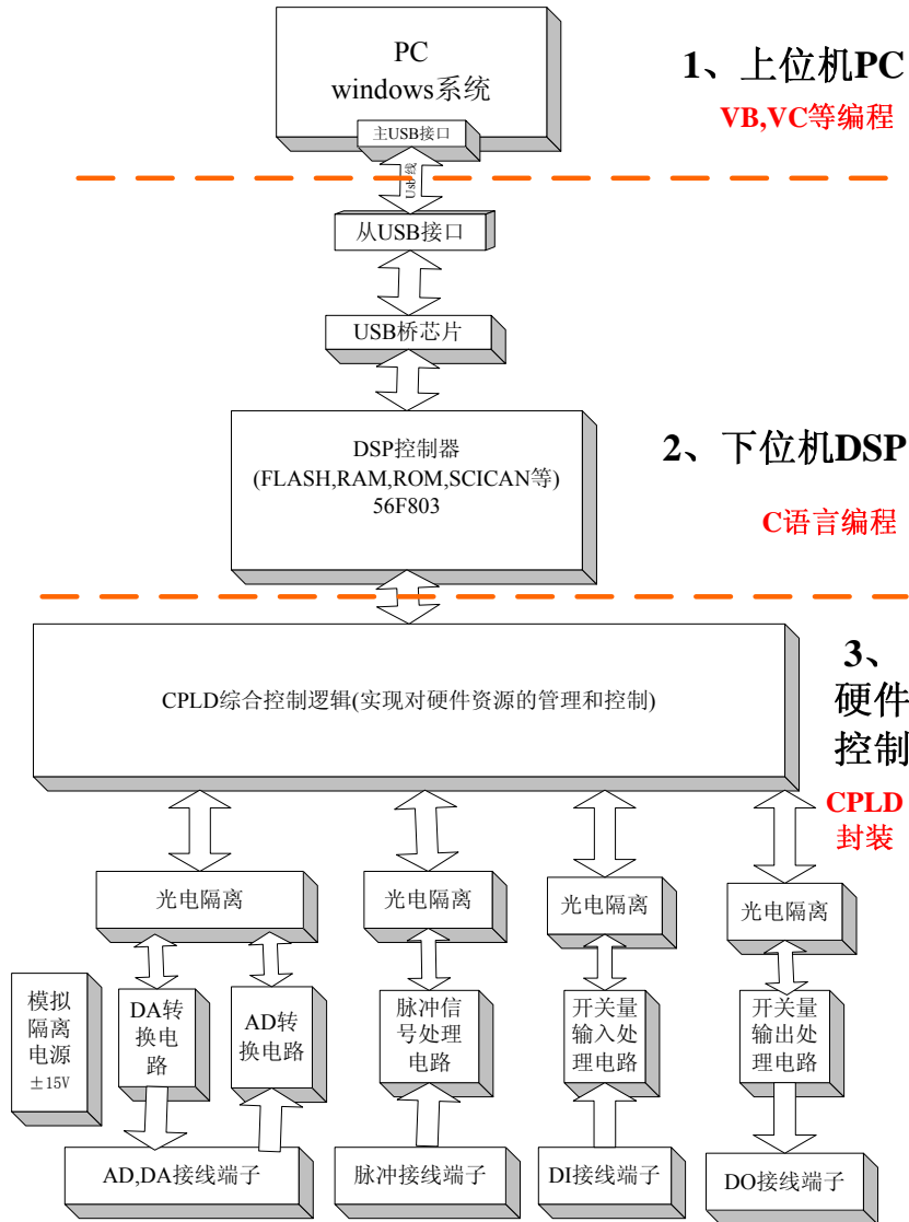
图 1 原理框图
