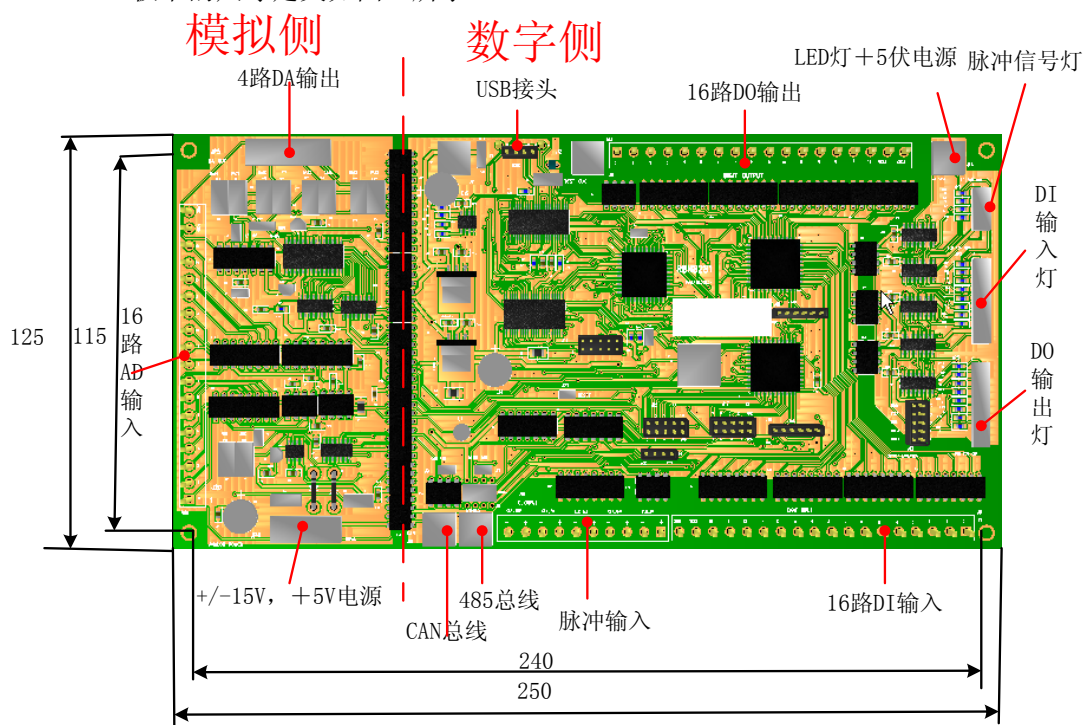
图 3 RBH8281 的尺寸
